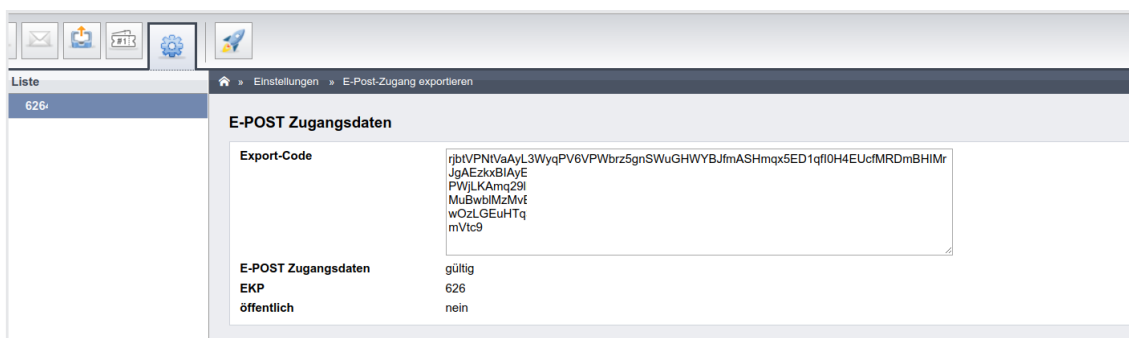
Abb. 416: Export Zugangsdaten
