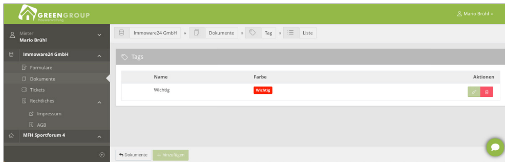
Abb. 17: Ansicht Tags
