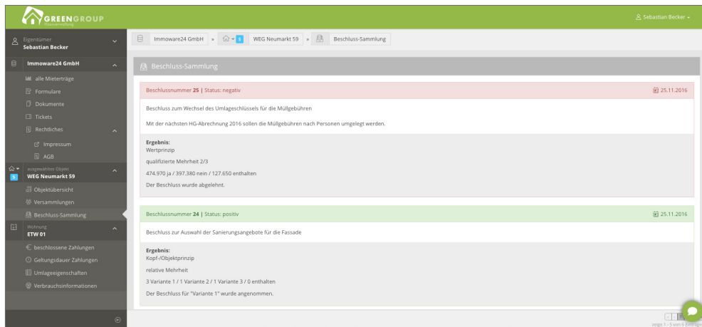
Abb. 33: Ansicht Beschluss-Sammlung
