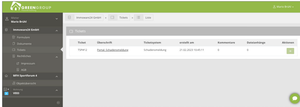
Abb. 20: Ansicht Tickets
