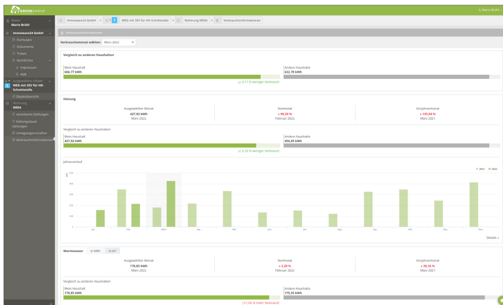
Abb. 32: Ansicht Verbrauchsinformationen
